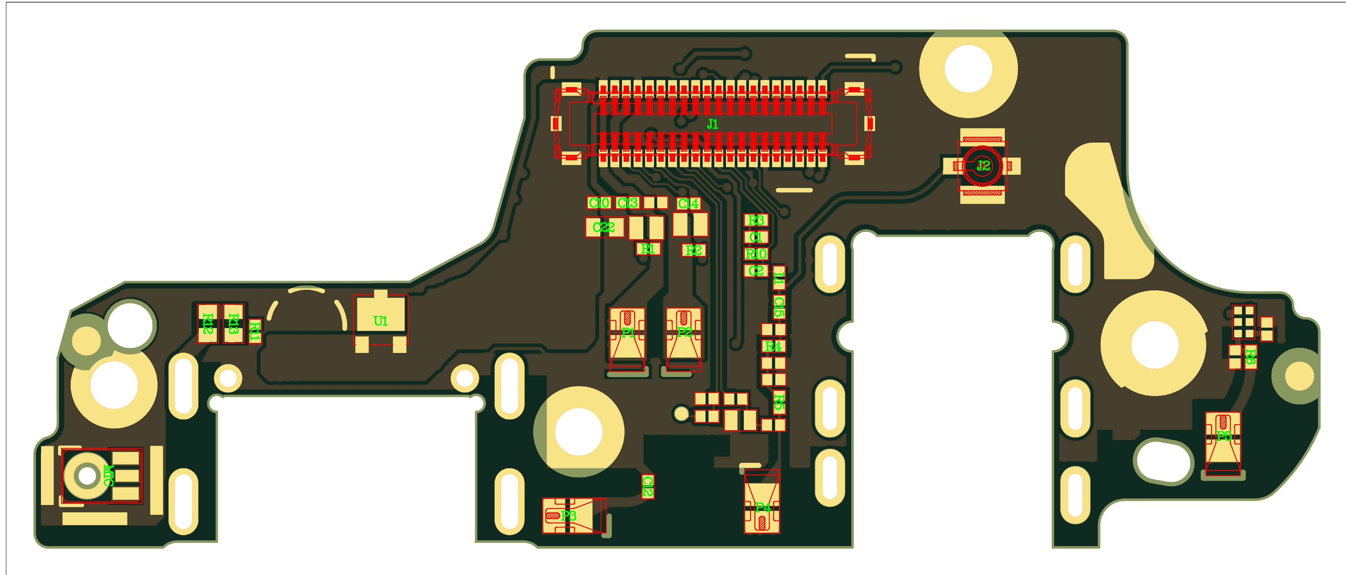
H M N T 9 S W C _ P C B - 正面元件位置图
