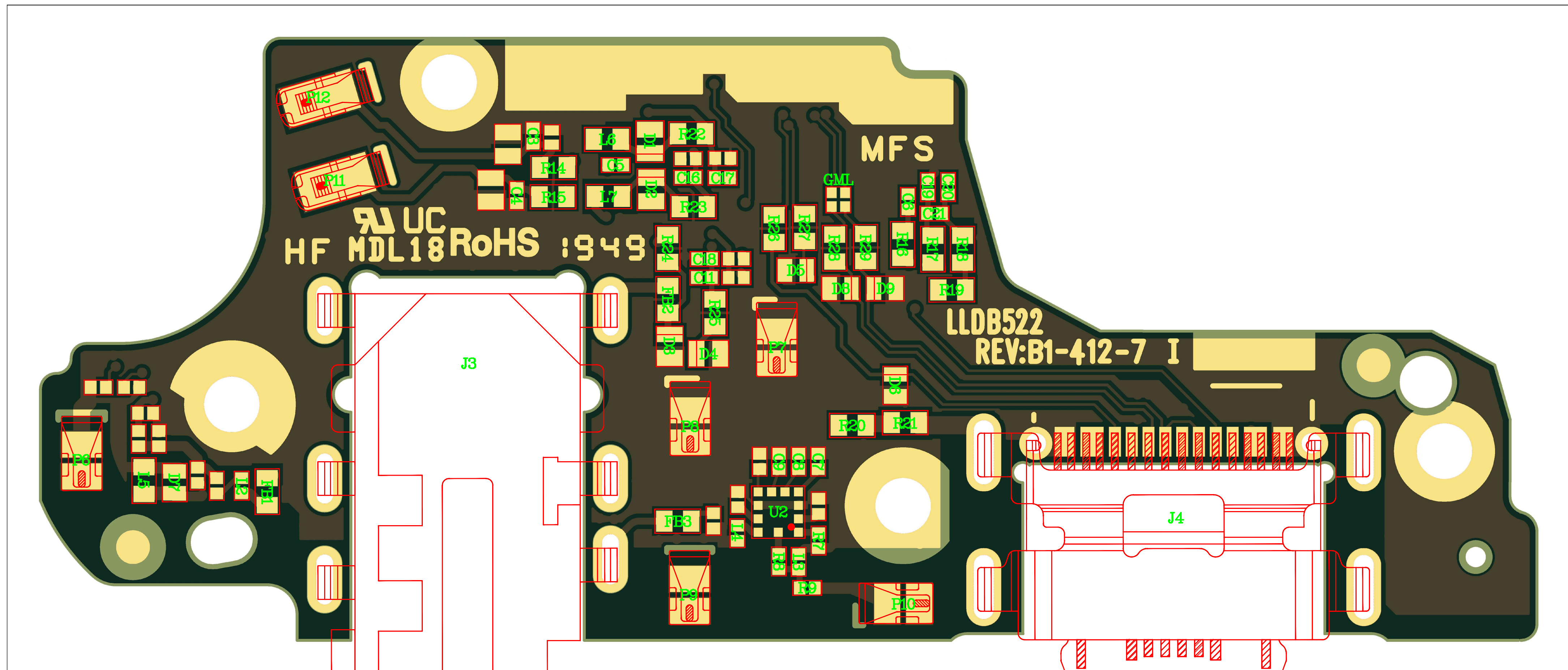
H M N T 9 S W C _ P C B - 反面元件位置图
